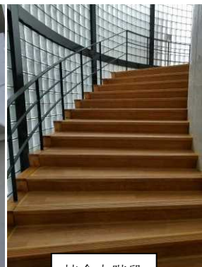
校舎内階段
